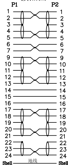
接点图
